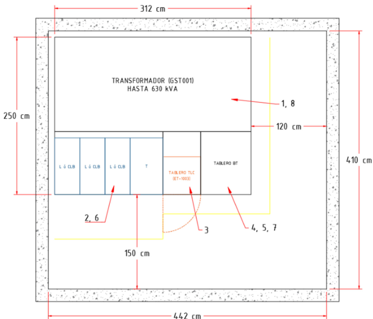
Figura 10. Vista planta
