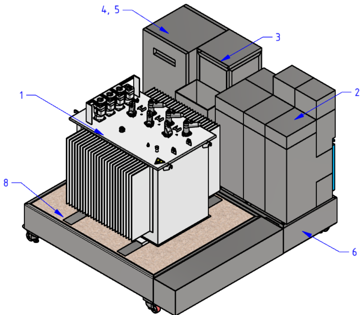
Figura 4. Vista isométrica posterior
