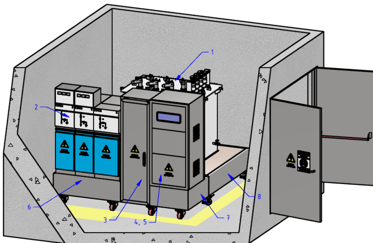
Figura 3. Vista corte dentro de recinto
