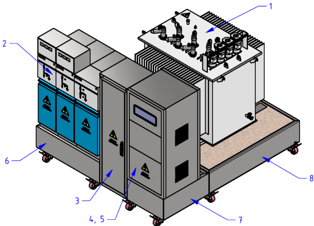
Figura 1. Vista isométrica frontal.
