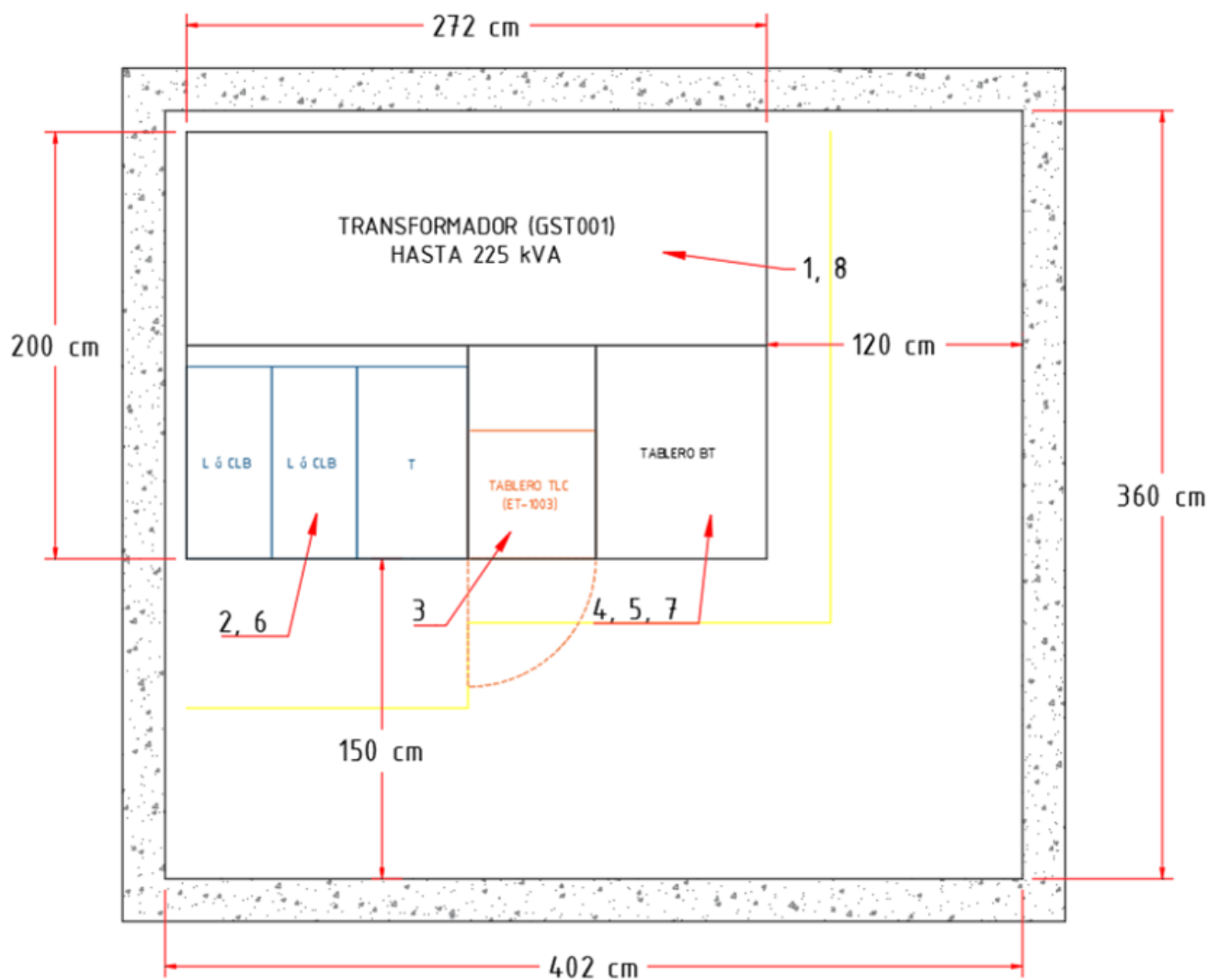
Figura 6. Vista planta
