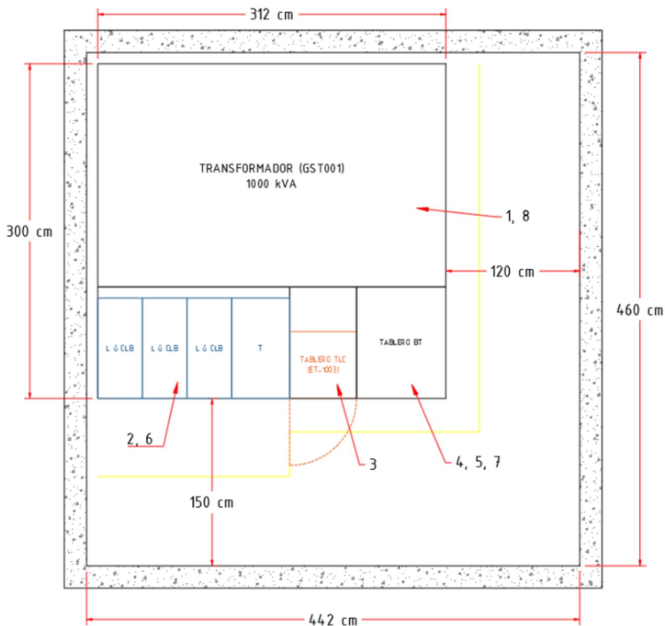
Figura 13. Vista planta
