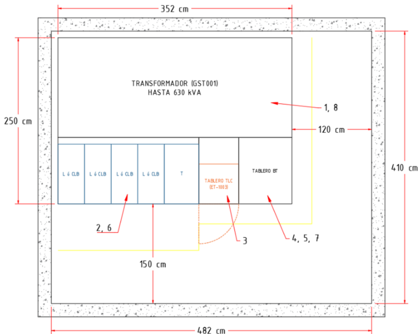
Figura 11. Vista planta
