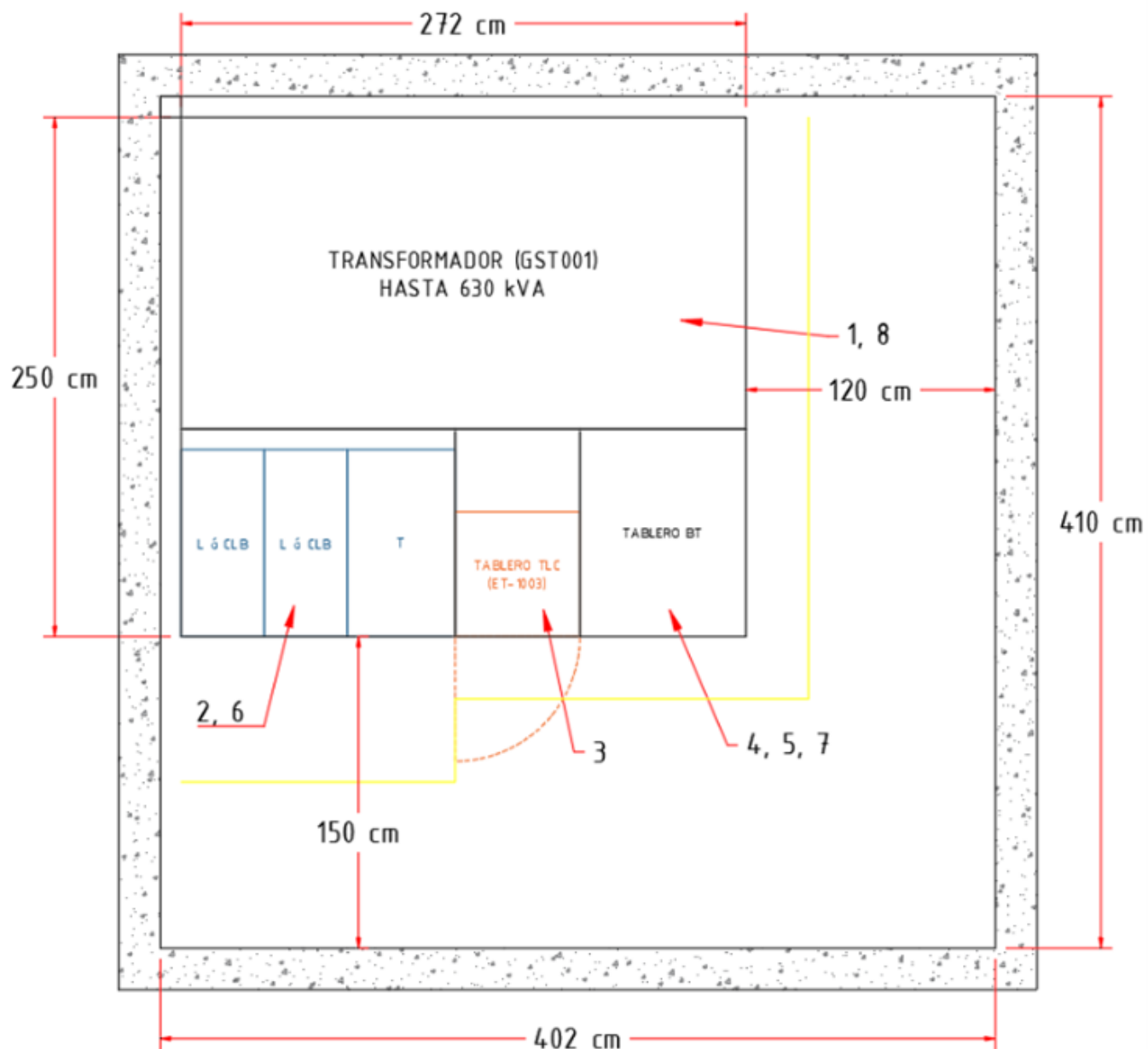
Figura 9. Vista planta
