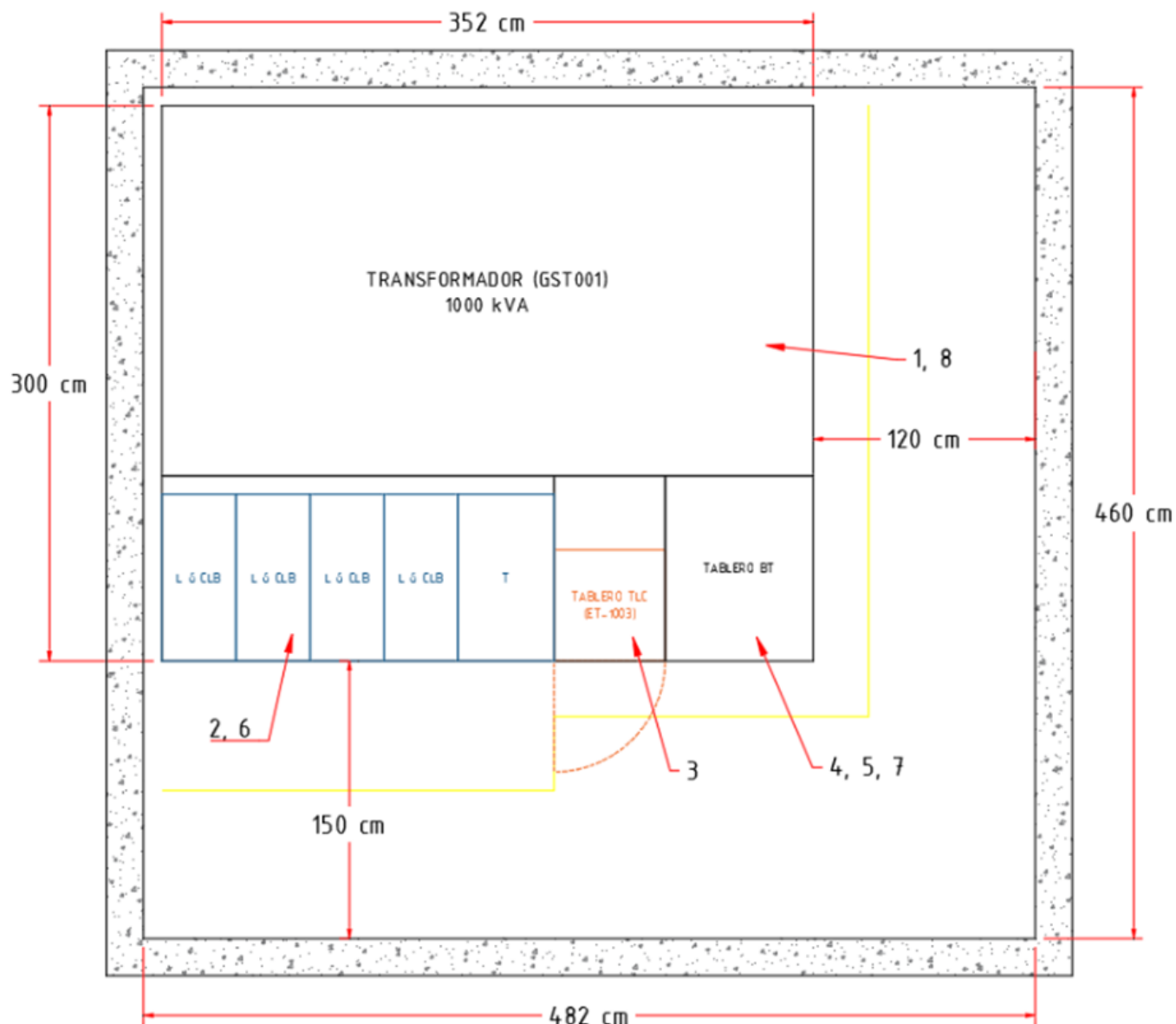
Figura 14. Vista planta
