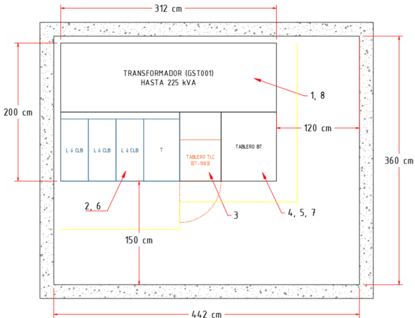
Figura 7. Vista planta
