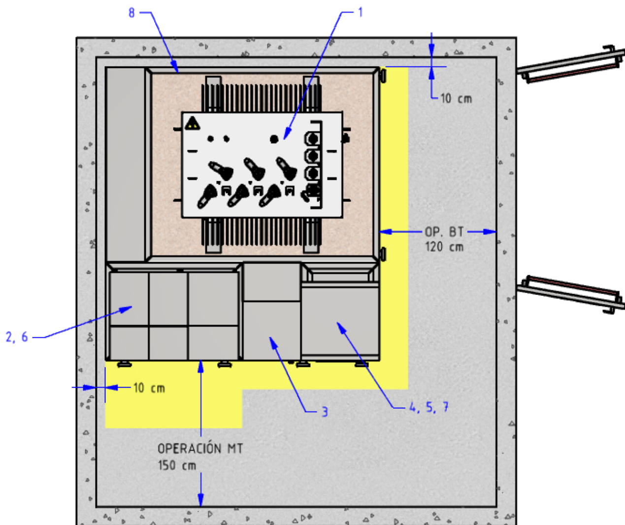
Figura 2. Vista planta.
