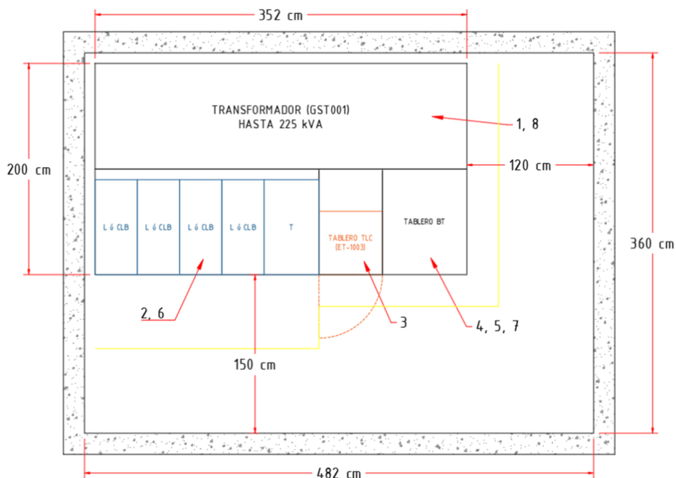
Figura 8. Vista planta
